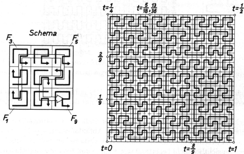
Figur 5 Näherungspolygon 3. Ordnung der Peano-Kurve vom Mäandertyp.
