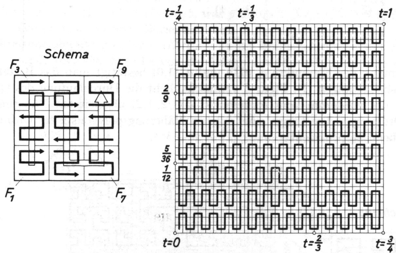
Figur 4 Näherungspolygon 3. Ordnung einer Peano-Kurve vom Serpentinertyp 111 111 111.
