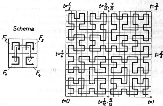
Figur 1 Näherungspolygon 4. Ordnung der Hilbertschen Peano-Kurve.
