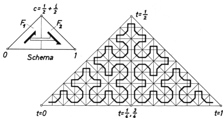
Figur 6 Näherungspolygon 7. Ordnung der Knoppschen Peano-Kurve.
