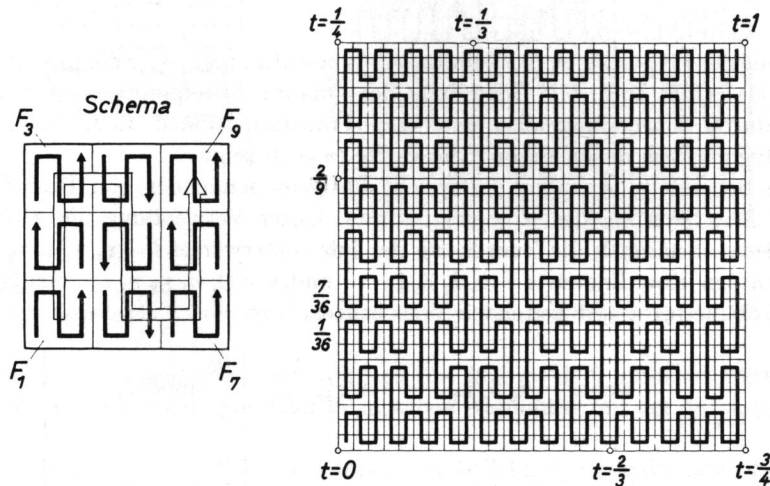
Figur 2 Näherungspolygon 3. Ordnung einer Peano-Kurve vom Serpentinertyp 000 000 000.
