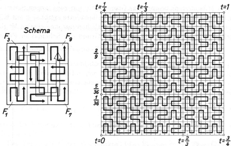
Figur 3 Näherungspolygon 3. Ordnung einer Peano-Kurve vom Serpentinertyp 010 101 010.
